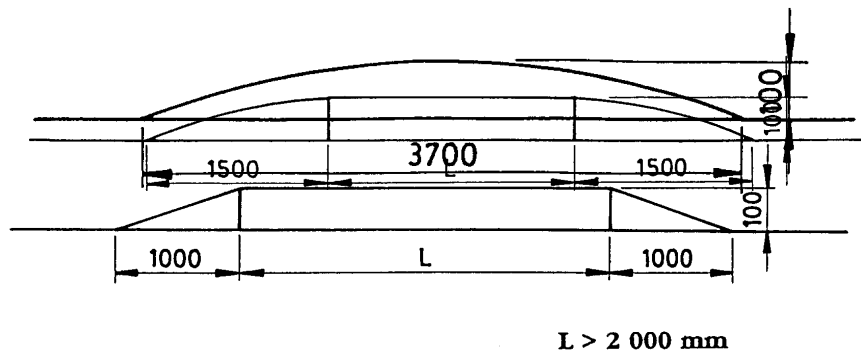
Rys. 1. Kształt i wymiary progów liniowych typu 1 (dla granicznej prędkości przejazdu 25-30 km/h) a. Próg listwowy typu 1
