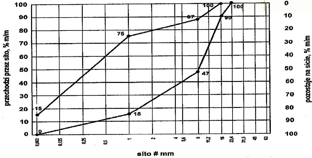
Uziarnienie mieszanki niezwiązanej 0/16 dla warstwy mrozoochronnej
