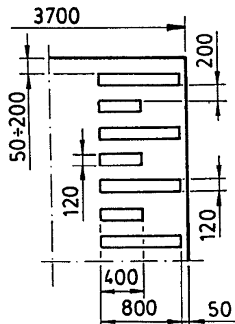
Rys. 2. Oznakowanie poziome
