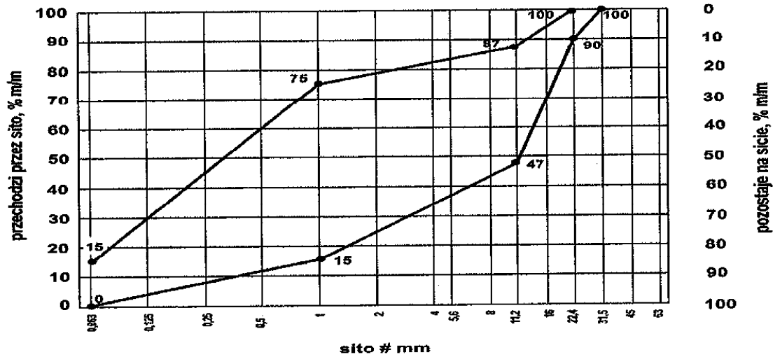
Uziarnienie mieszanki niezwiązanej 0/22,4 dla warstwy mrozoochronnej
